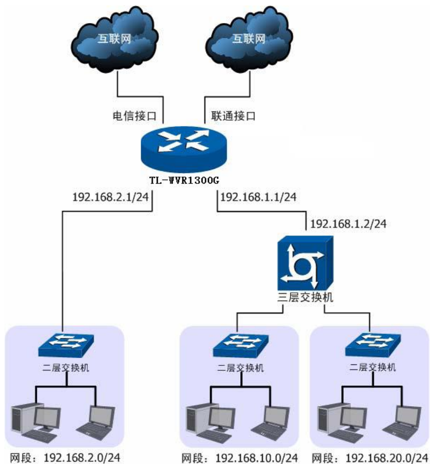
图 4-36 NAPT功能组网应用
