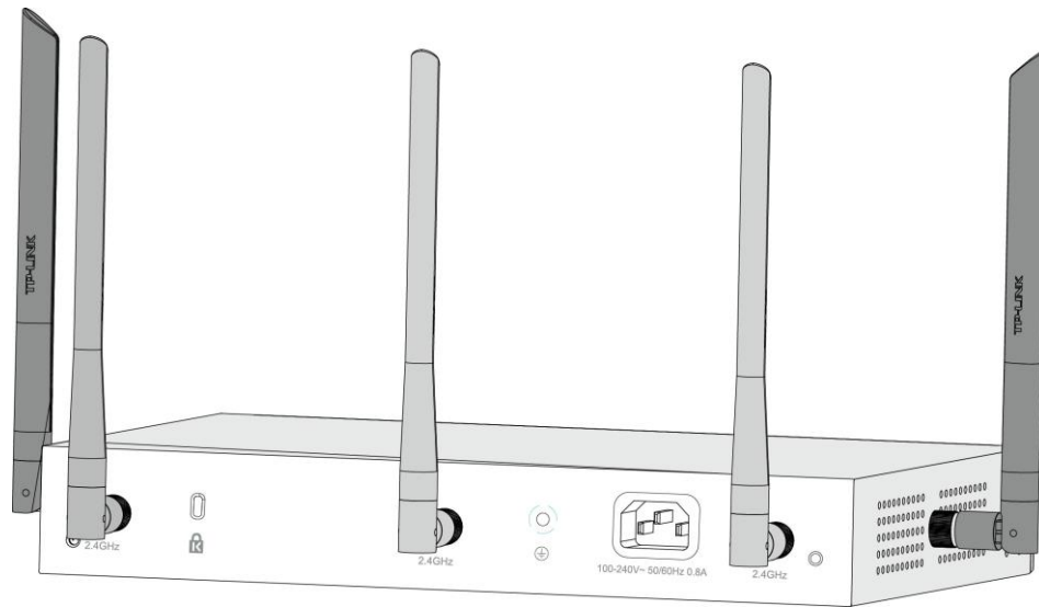
图 2-2 TL-WVR1300G后面板示意图
