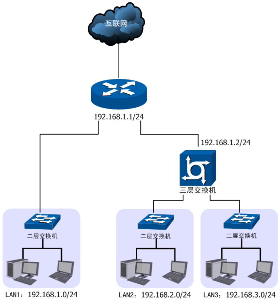
图 4-51 静态路由功能组网应用
